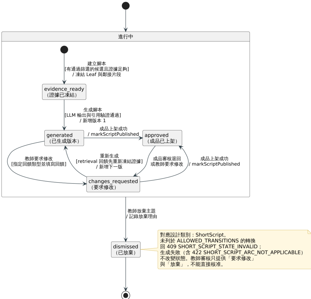
圖 7-4-7 短影音腳本狀態機圖
