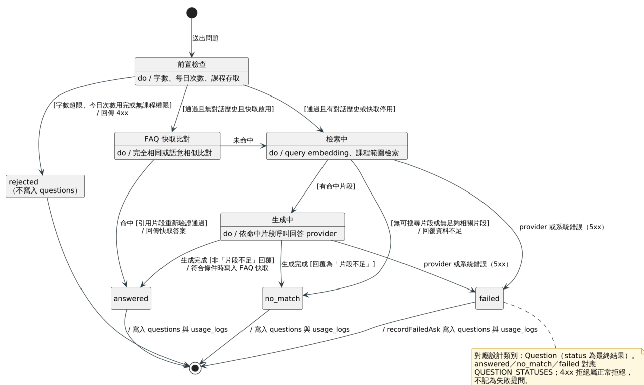
圖 7-4-4 QA 提問狀態機圖
