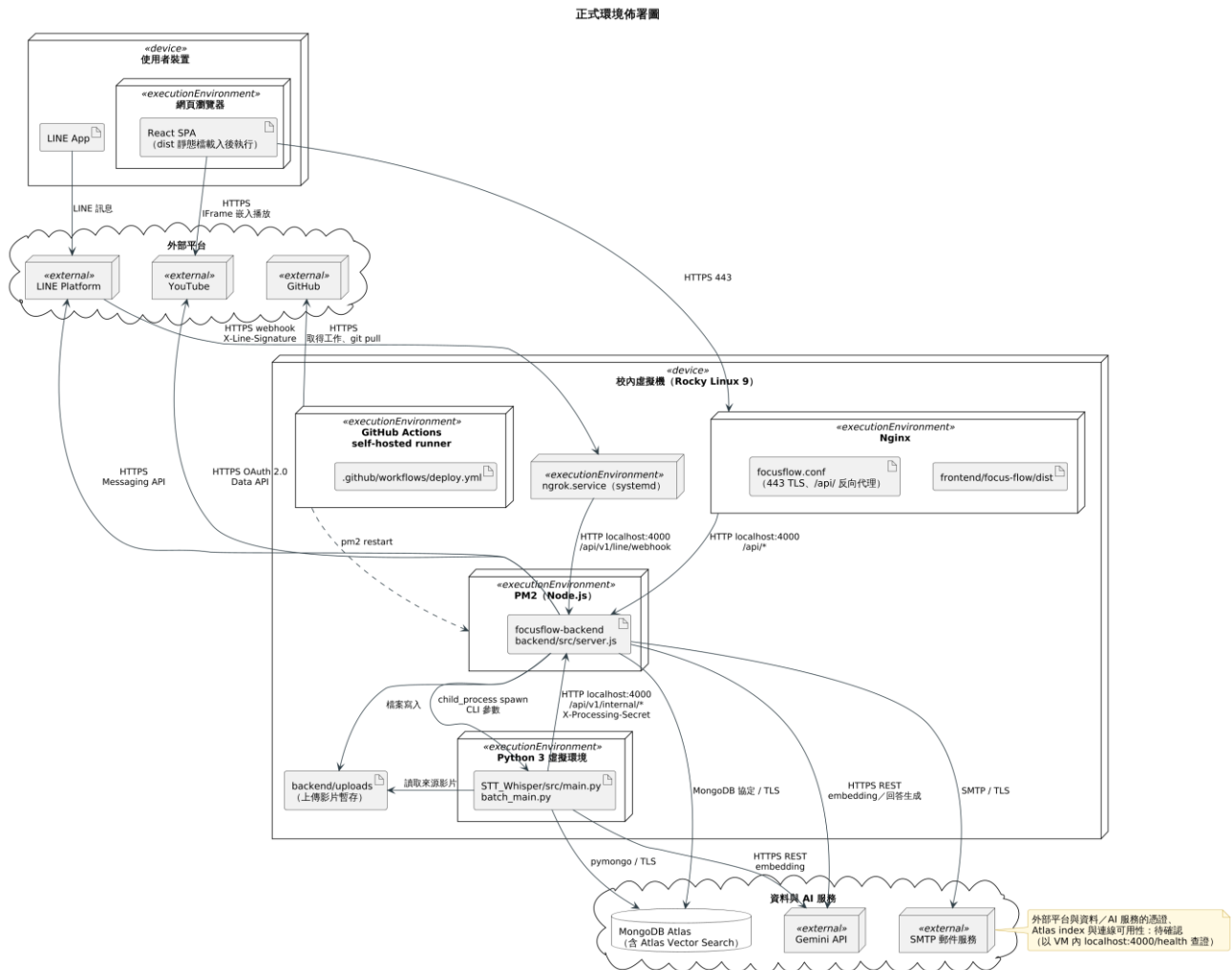
圖 7-1-1 正式環境佈署圖
